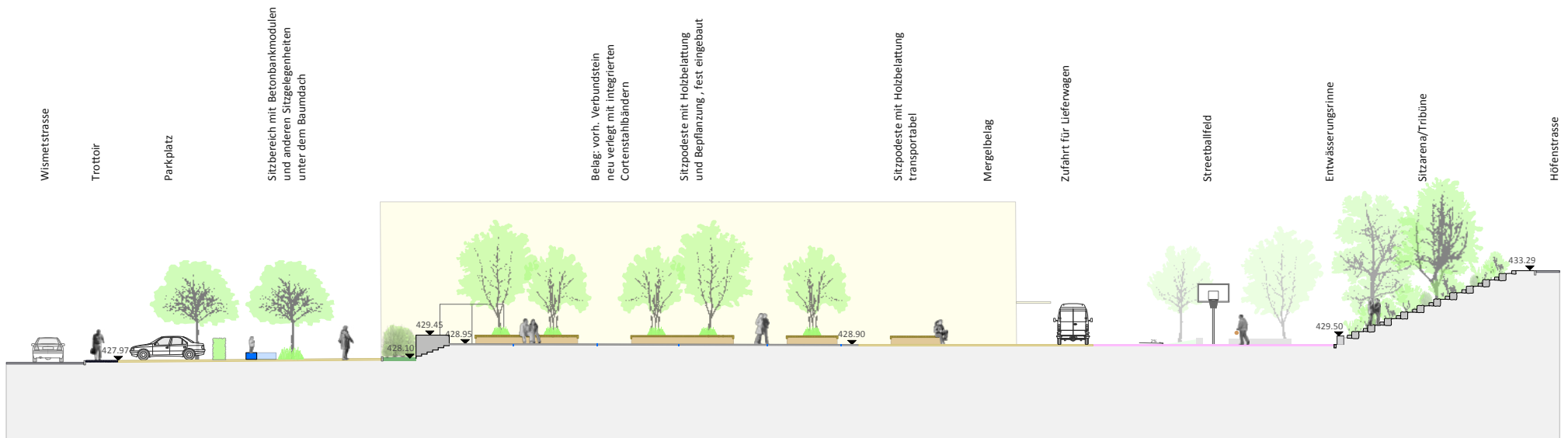
Schnitt A-A'
