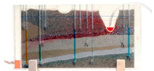
Infiltration aus einem verunreinigten Fluss ins Grundwasser.
